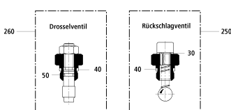
Ausführung bei Kolbenstangen- \varnothing 50, 63 und 80 mm
